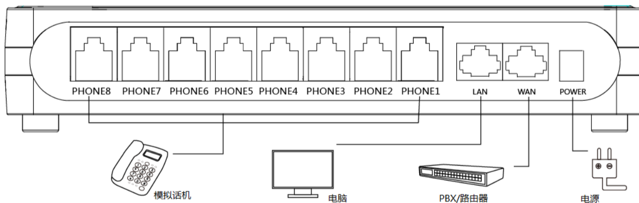
网络接口图
